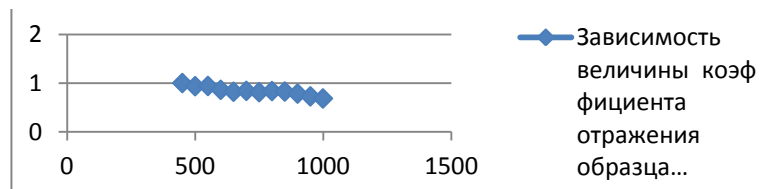
Рис. 1- Зависимость величины коэффициента отражения образца \text{Bi}_{0,6}\text{Sb}_{1,4}\text{Te}_3 + 2\% \text{Bi}_2\text{Se}_3 от длины волны зондирующего электромагнитного излучения
